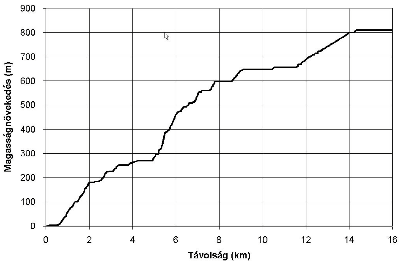
Magasságnövekedés profil
